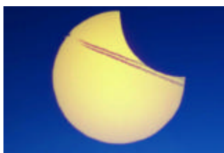
Bildnummer: so027-03 Ringförmige Sonnenfinsternis 3.10.2005, Sierra de Guadarrama nordwestlich von Madrid, Spanien. Partielle Phase mit Kondensstreifen eines Flugzeuges © Bernd Koch © Astrofoto/Bernd Koch
