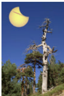
Bildnummer: so027-04 Ringförmige Sonnenfinsternis 3.10.2005, Sierra de Guadarrama nordwestlich von Madrid, Spanien. Partielle Phase mit Kondensstreifen eines Flugzeuges, Bäume im Vordergrund (Fotomontage) © Bernd Koch © Astrofoto/Bernd Koch
